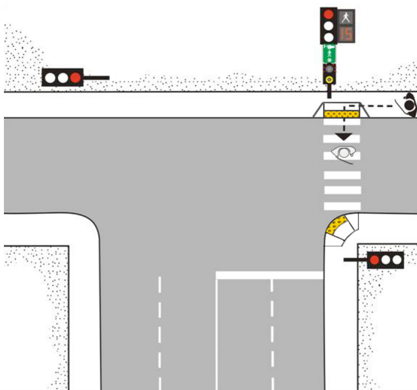
Croquis 20 : Position du bouton d'appel – Intersection en T
