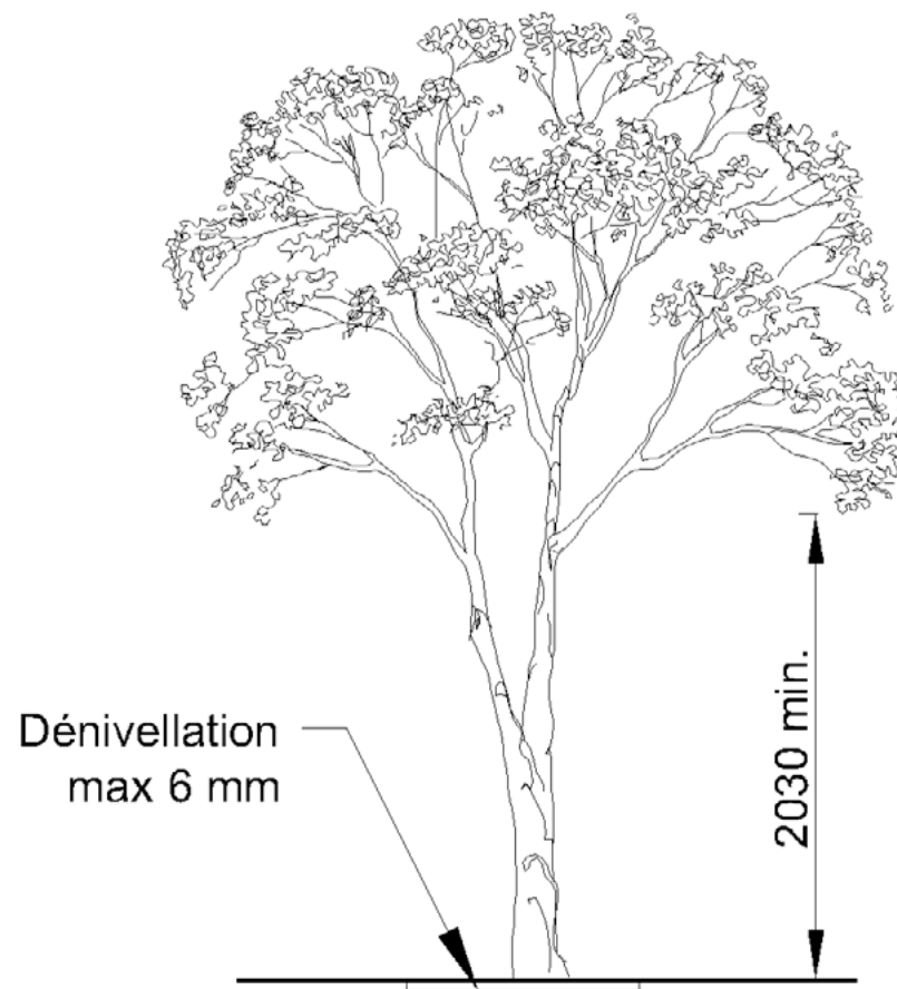
Croquis 5 : Zone de plantation au même niveau que le corridor piétonnier
