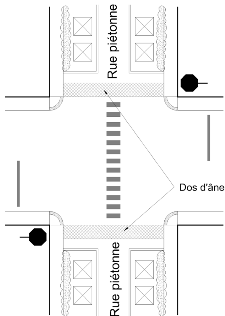
Croquis 5 : Intersection d'une rue piétonne et d'une rue de circulation automobile munie d'arrêts
