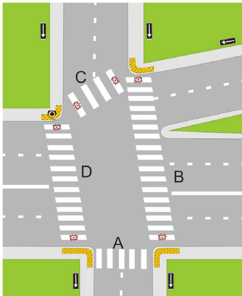
Croquis 15 : Intersection à branches multiples, besoin de signaux sonores aux passages B, C, D
