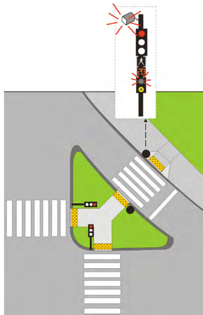
Croquis 7b : Passage pour piétons au centre de la bretelle, aménagé avec signaux sonores et trajectoires définies sur l'îlot
