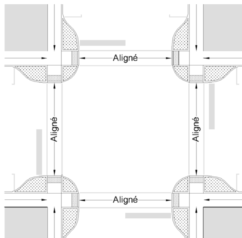
Croquis 13 : Aménagement de saillies sur les deux axes et aux quatre coins
